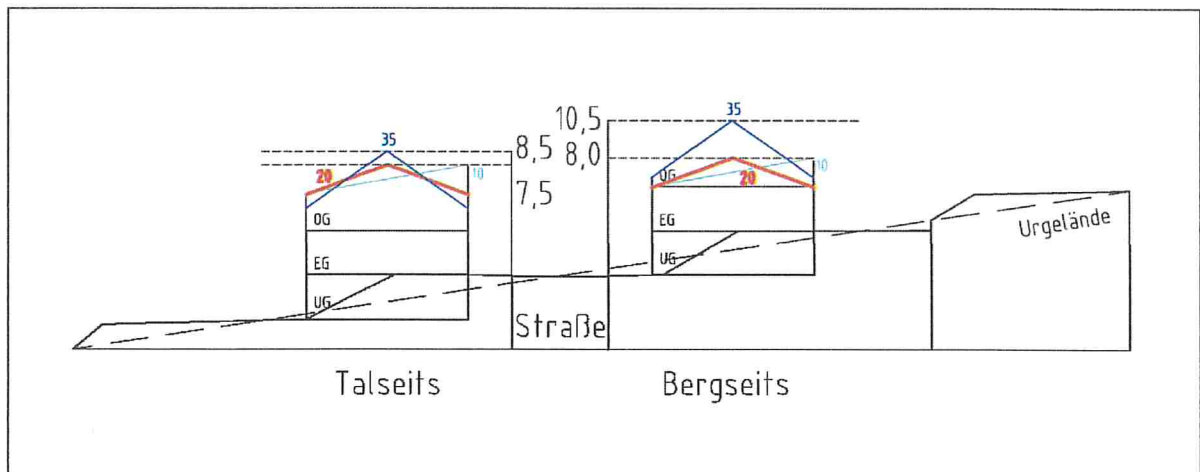
Abb. 1: Prinzipskizze Gebäudehöhe und Bezugspunkte
